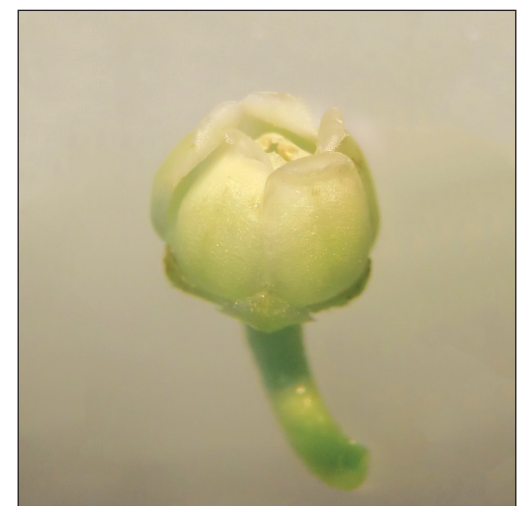
Rinorea niccolifera Fernando, sp. nov.
